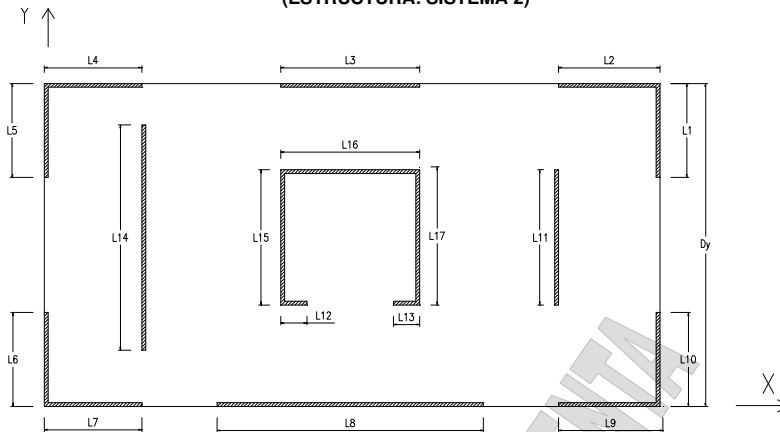
FIGURA 2 SISTEMA DE MUROS ORTOGONALES (X,Y) (ESTRUCTURA: SISTEMA 2)
