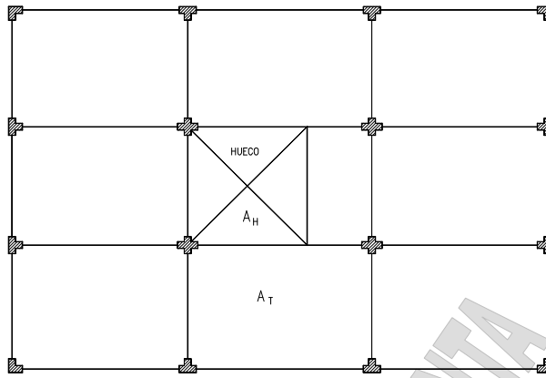
FIGURA 8 EJEMPLO DISCONTINUIDAD EN LOSAS
